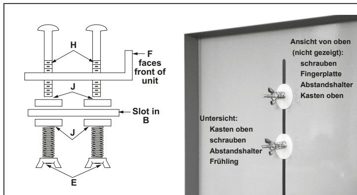
FIGUR 3 Schiebevorrichtungsbaugruppe
