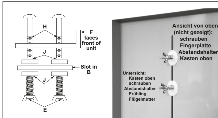
FIGUR 3 Schiebevorrichtungsbaugruppe
